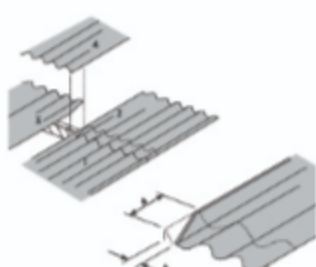
a = recobrimento longitudinal adotado b = recobrimento lateral = 1/4 de onda (50 mm) ou 1/3 de onda (280 mm) para espessuras de 6 e 8 mm
